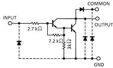
ULN2003APG/AFWG
